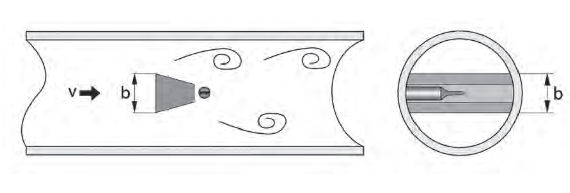
Рисунок 8-1: Принцип действия
