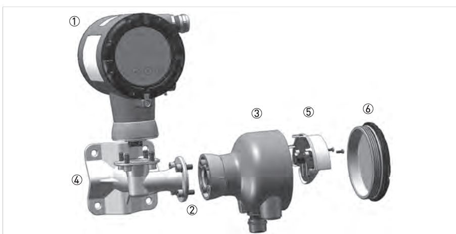
Рисунок 7-4: Модуль преобразователя сигналов отдельного исполнения в разобранном виде
